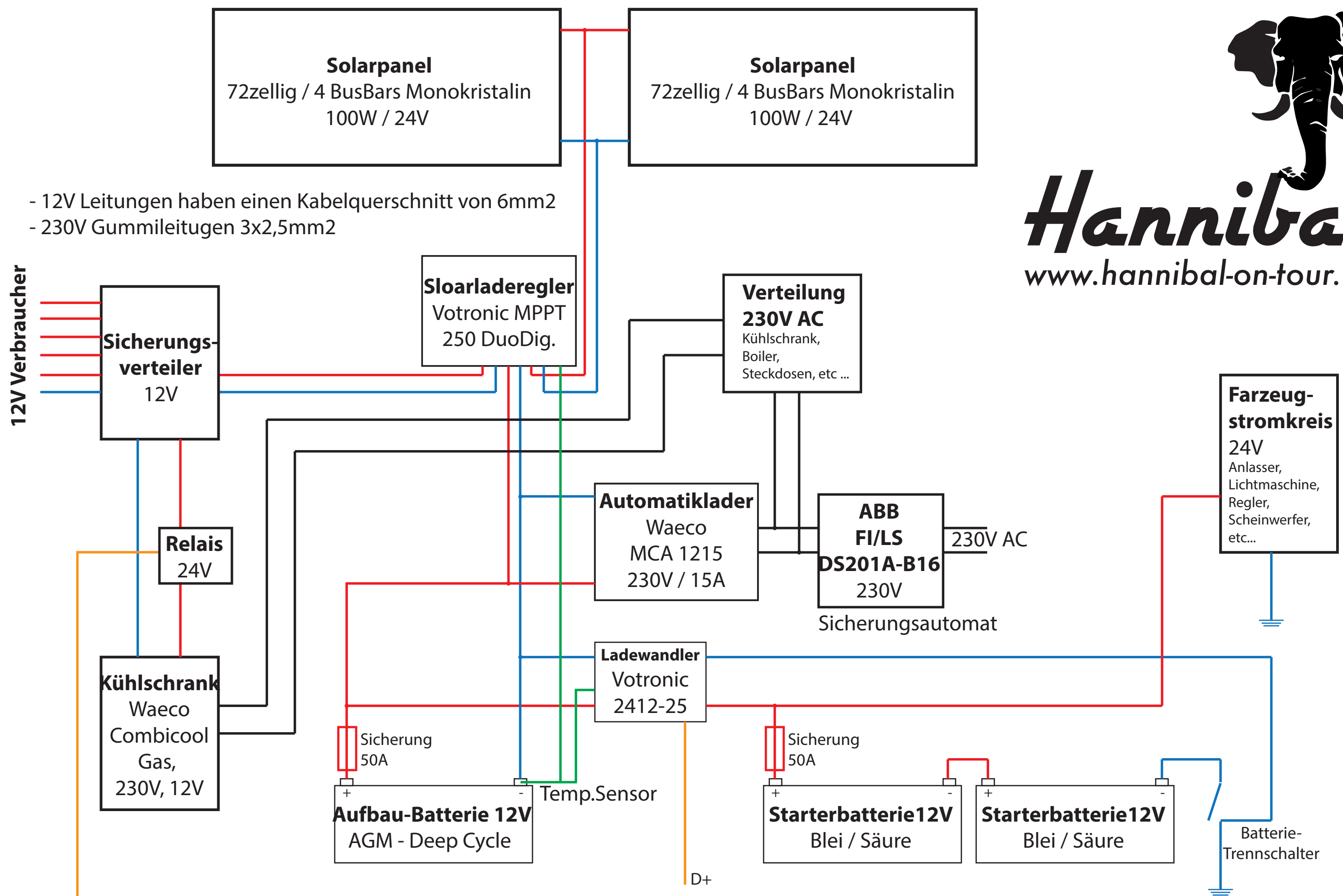
Stromlaufplan Wohnmobilausbau MB L508DG- schematische Darstellung - 24V Bordstromkreis / 12V Wohnstromkreis Kontakt: info@hannibal-on-tour.de - http://www.hannibal-on-tour.de - KEINE HAFTUNG FÜR EVENTUELLE FEHLER!
